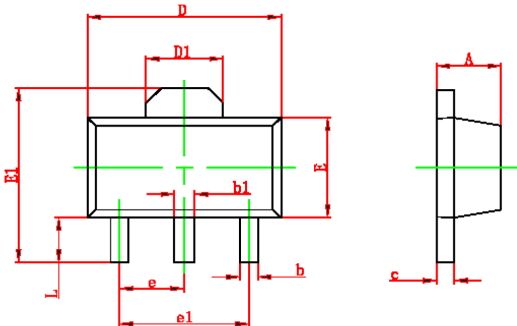
SOT-89-3 封装尺寸图
