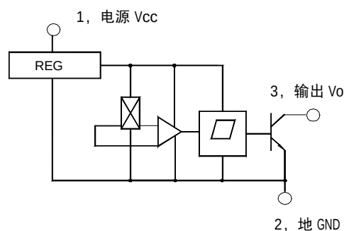
功能方框图
