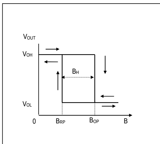
磁电转换特性图
