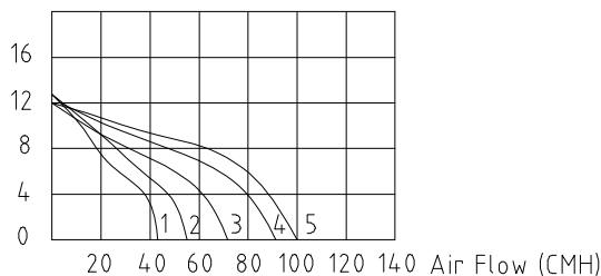
ΔP(PA) 230V/50Hz
