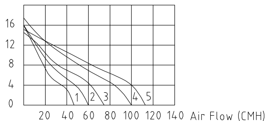
ΔP(PA) 120V/60Hz
