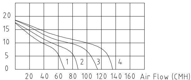
ΔP(PA) 230V/50Hz
