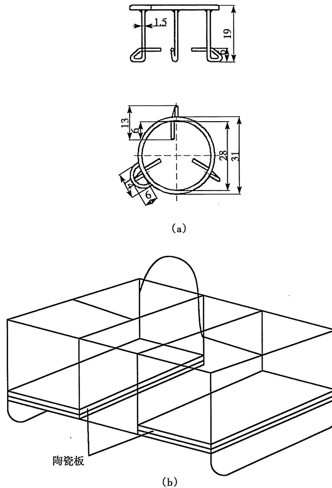
图2 坩埚架示意图(单位为毫米)
