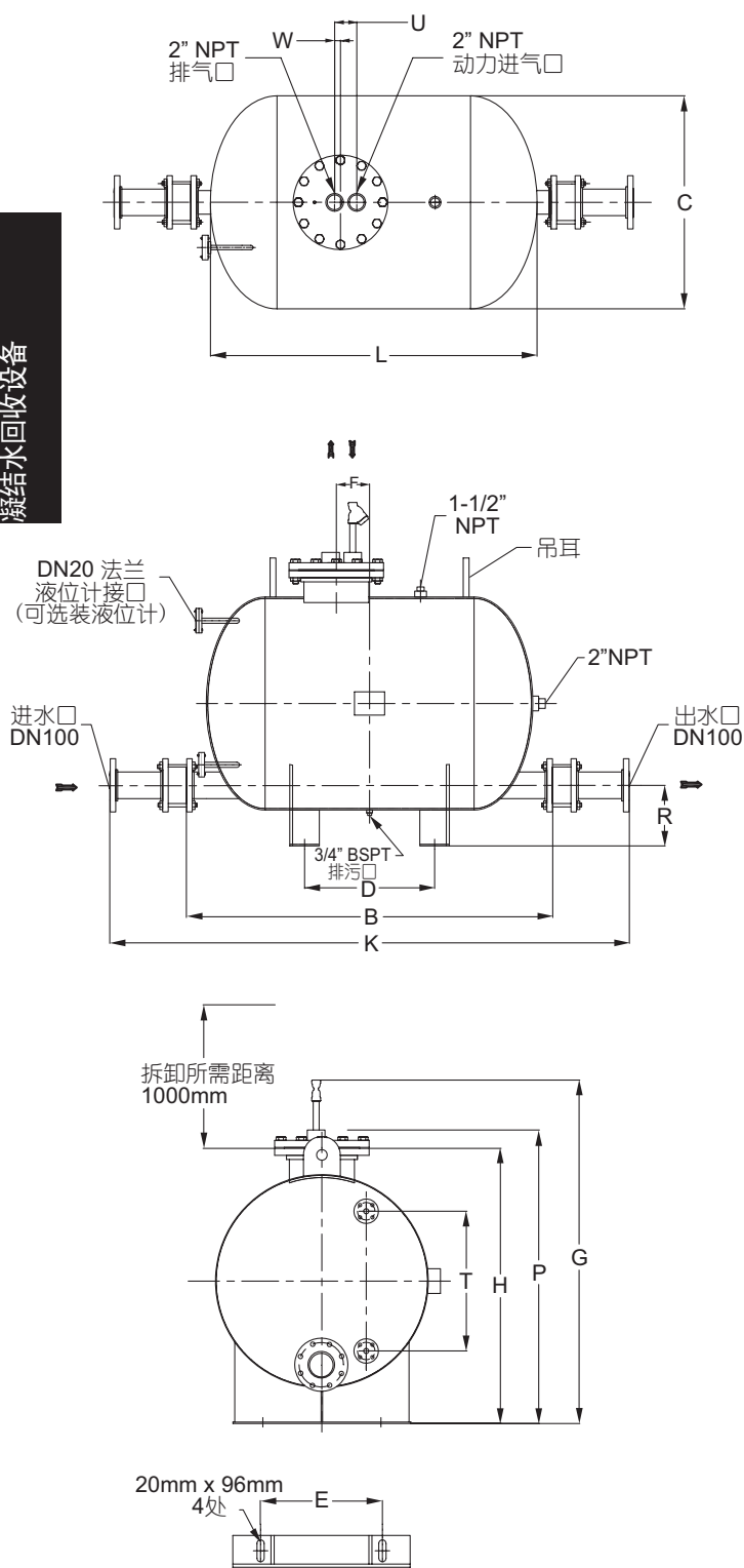
PT-516大排量凝结水回收泵物理数据
