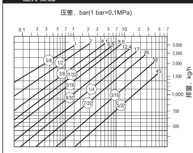
316 型排量图
