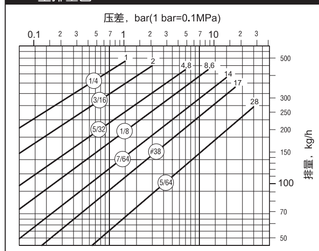
313 型排量图
