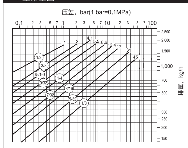
315 型排量图
