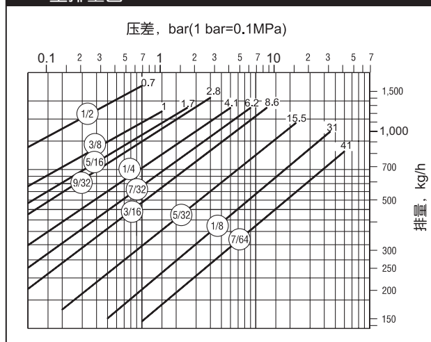
314 型排量图
