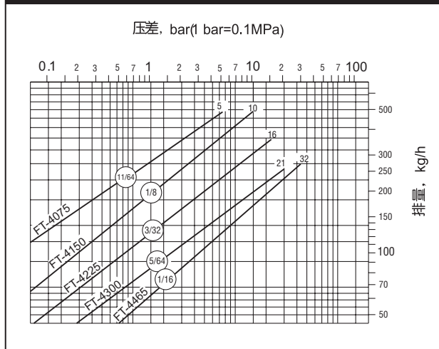
FT-4000 系列排量图
