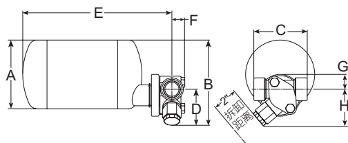
FT-4000系列带TVS-4000疏水阀站
