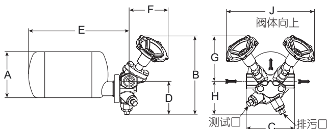
FT-4000系列带TVS-4000疏水阀站
