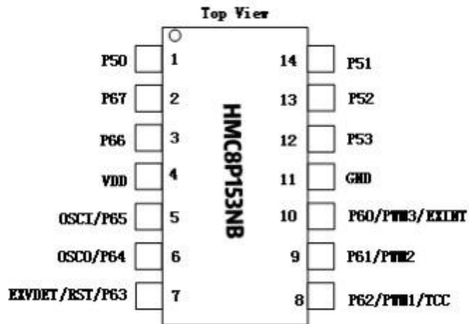
HMC8P153NB-14PIN 脚位图
