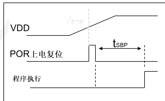
图 10: 上电复位时序图
