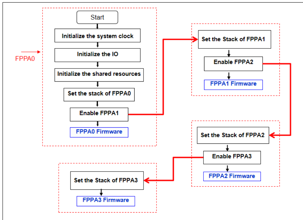
图 11: 开机流程
