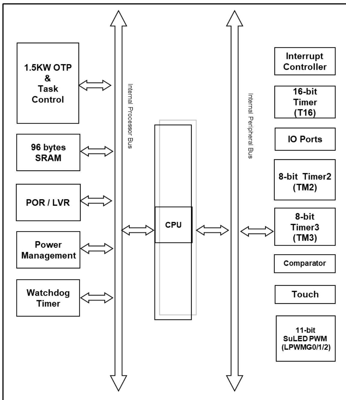
图 1: PMS160 系统方框图
