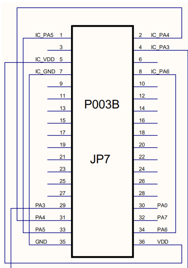
图 28: 使用 P003B 时，PMS160-S08B JP7 跳线原理图
