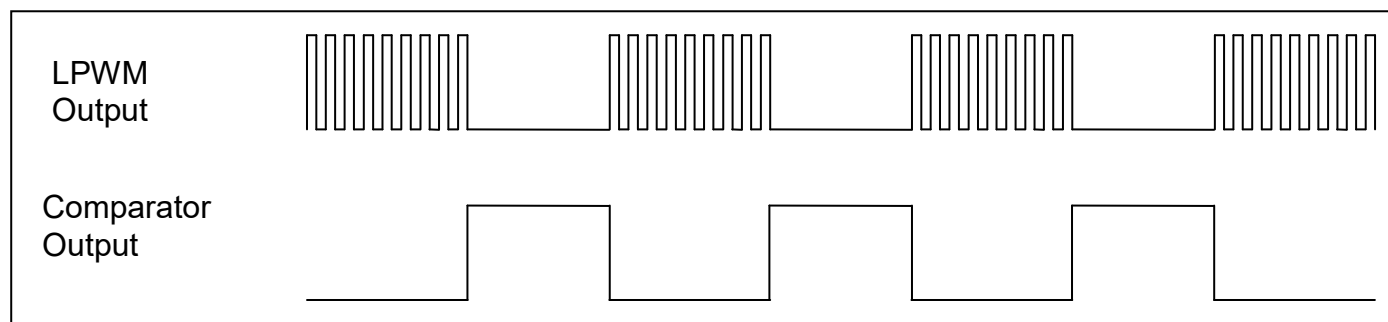
图 20: 比较器控制 LPWM 波形的输出
