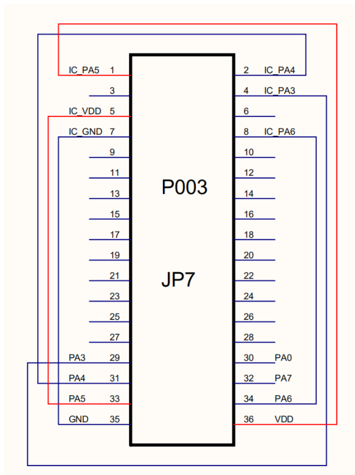
图 26: 使用 P003 时, PMS160-S08B JP7 跳线原理图
