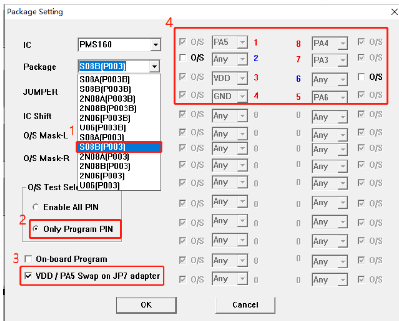
图 25: PMS160-S08B 在 P003 转档配置
