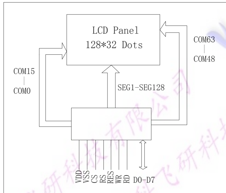
图2: 12832C3G图像点阵型液晶模块的电路框图
